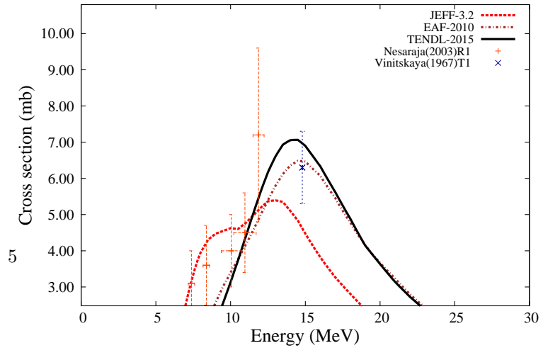
^{72}\text{Ge}(n,a)^{69g}\text{Zn}
