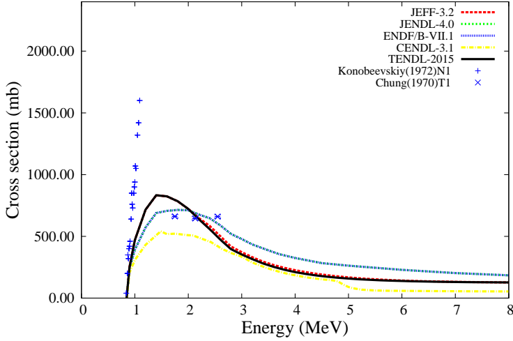
^{72}\text{Ge}(n,g)^{73}\text{Ge}
