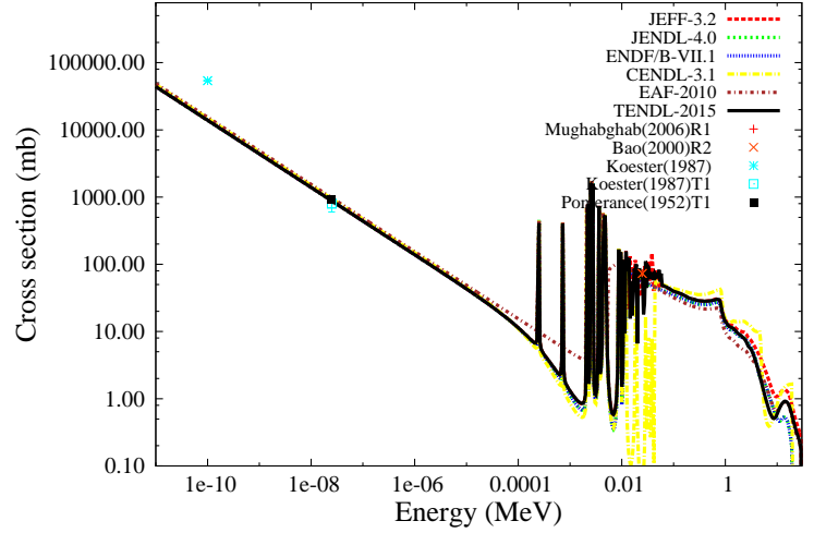
^{72}\text{Ge}(n,g)^{73}\text{Ge}
