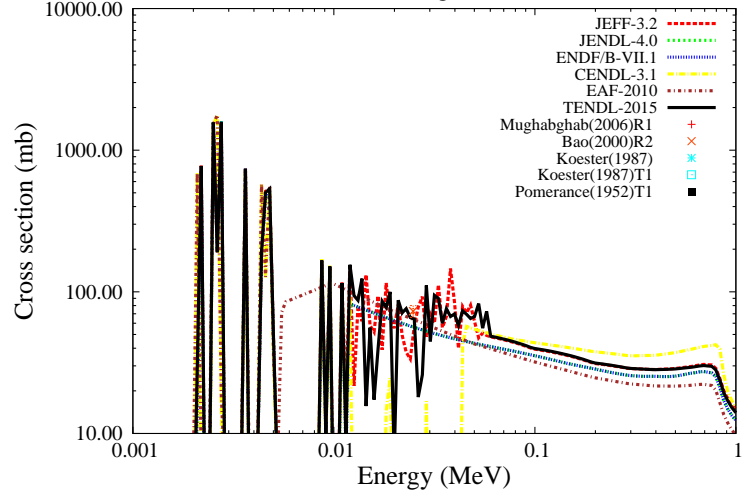
^{72}\text{Ge}(n,a)^{69g}\text{Zn}
