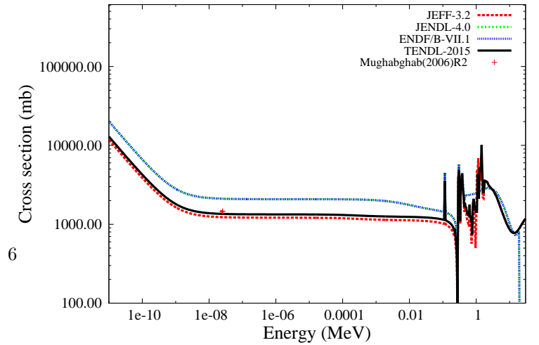
^{34}\text{S}(n,\text{el})
