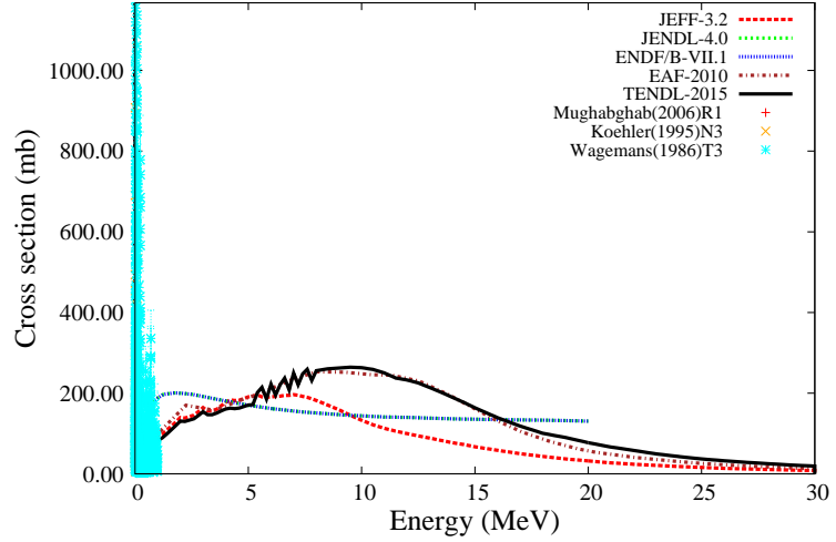
^{34}\text{S}(n,\text{tot})
