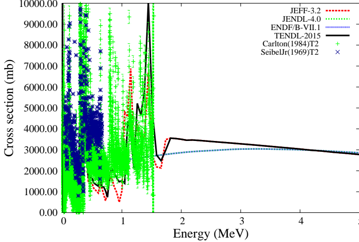
^{34}\text{S}(n,\text{tot})
