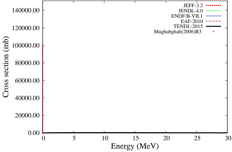
^{34}\text{S}(n,\text{tot})
