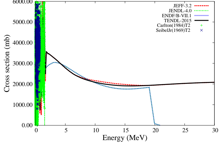
^{34}\text{S}(n,\text{el})
