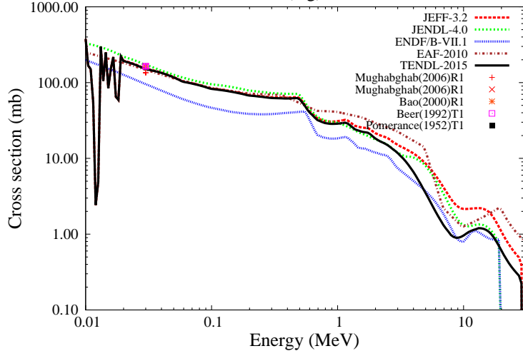
^{76}\text{Se}(n,g)^{77}\text{Se}
