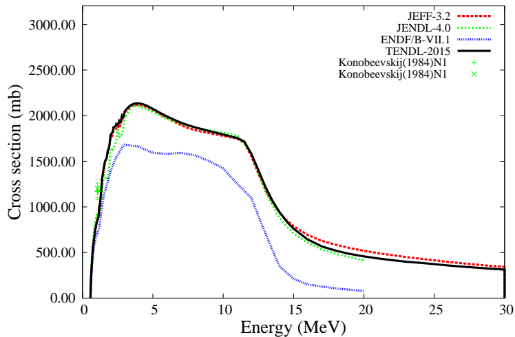
^{76}\text{Se}(n,n_1')^{76}\text{Se}
