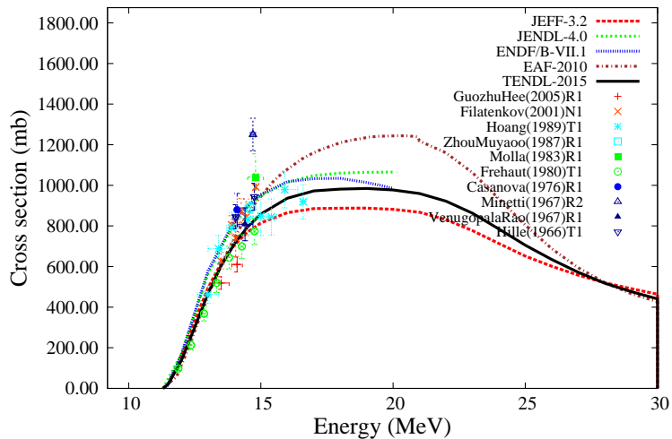
^{76}\text{Se}(n,g)^{77}\text{Se}
