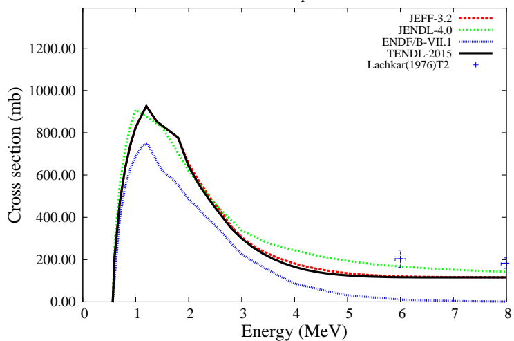
^{76}\text{Se}(n,g)^{77}\text{Se}
