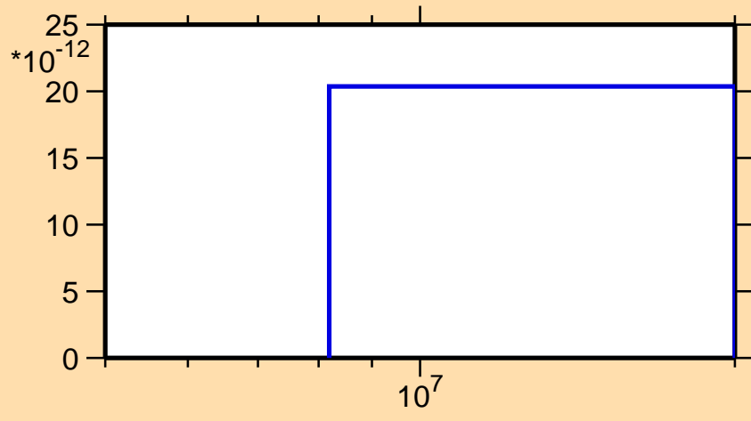
\sigma vs. E for ^{67}\text{As} (mt 34)
