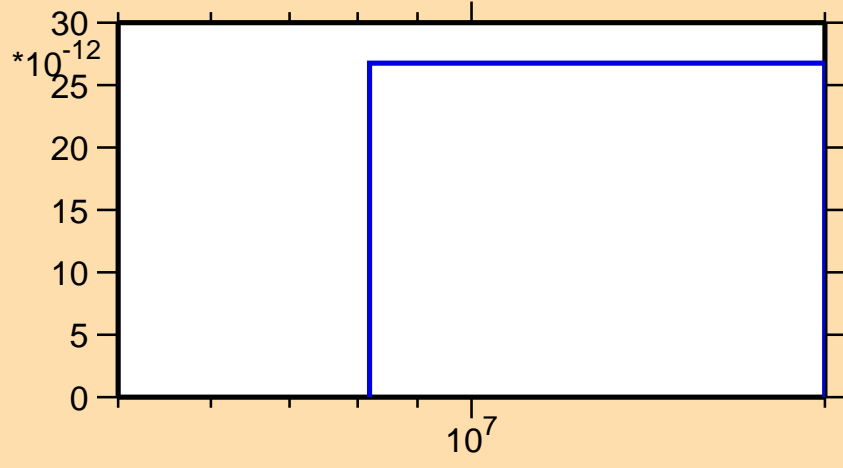
\sigma vs. E for ^{242}\text{Es} (mt 45)
