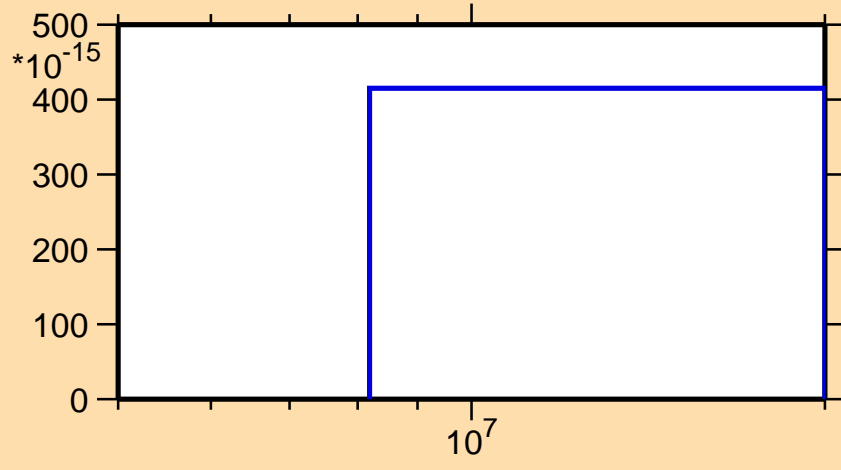
\sigma vs. E for ^{242}\text{Es} (mt 34)
