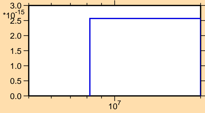
\sigma vs. E for ^{253}\text{Es} (mt 42)
