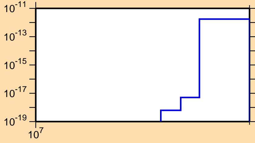
\sigma vs. E for ^{257}\text{Es} (mt 42)
