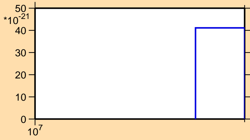
\sigma vs. E for ^{206}\text{Fr}(\text{mt } 42)
