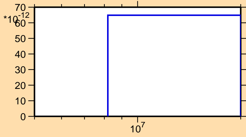
\sigma vs. E for ^{63}\text{Ga}(\text{mt } 34)
