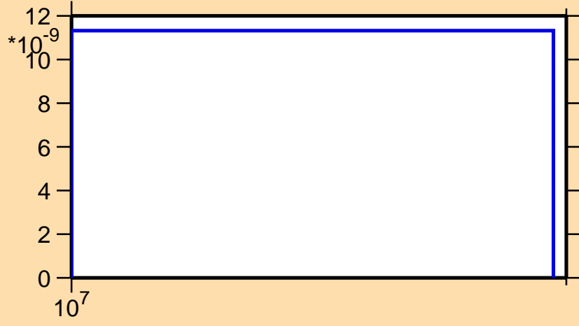
\sigma vs. E for ^{64}\text{Ga} (mt 34)
