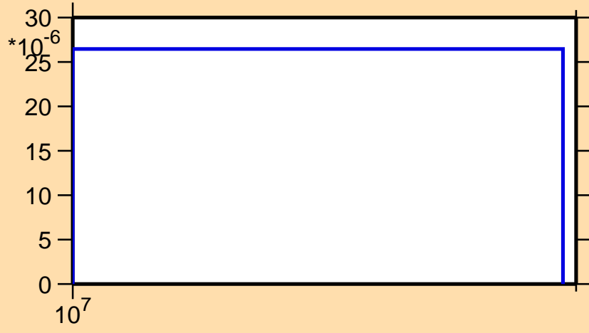
\sigma vs. E for ^{64}\text{Ga} (mt 45)
