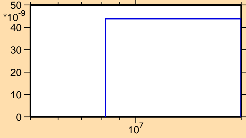
\sigma vs. E for ^{142}\text{Gd}(\text{mt } 45)
