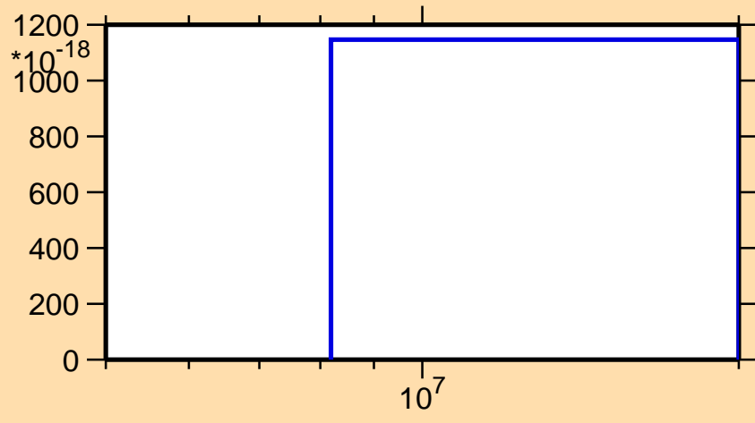
\sigma vs. E for ^{146}\text{Gd}(\text{mt } 34)
