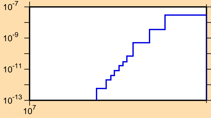
\sigma vs. E for ^{148}\text{Gd}(\text{mt } 45)
