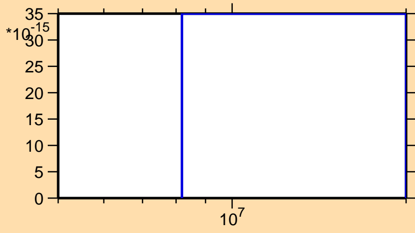
\sigma vs. E for ^{148}\text{Gd}(\text{mt } 34)
