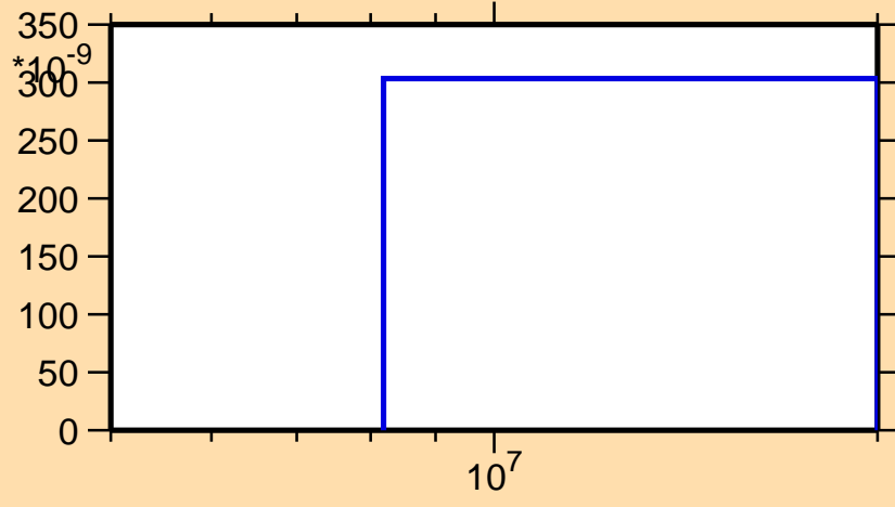
\sigma vs. E for ^{64}\text{Ge}(\text{mt } 45)
