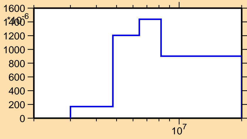
\sigma vs. E for ^{64}\text{Ge}(n,n\text{cont.})
