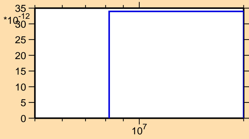
\sigma vs. E for ^{64}\text{Ge}(\text{mt } 34)
