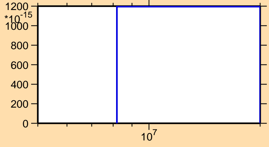
\sigma vs. E for ^{73}\text{Ge}(n,nt)
