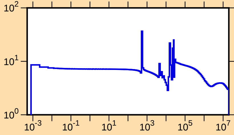
\sigma vs. E for ^{76}\text{Ge}(n,\text{tot.})
