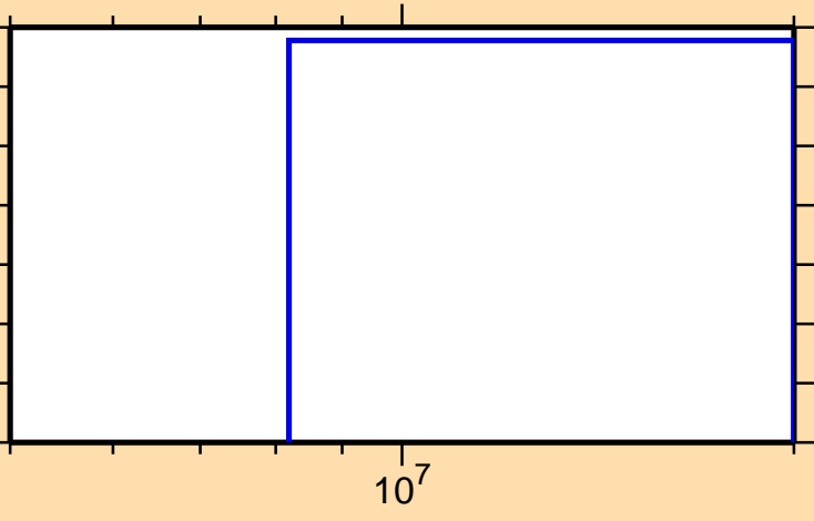
\sigma vs. E for ^{73}\text{Kr}(\text{mt } 45)
