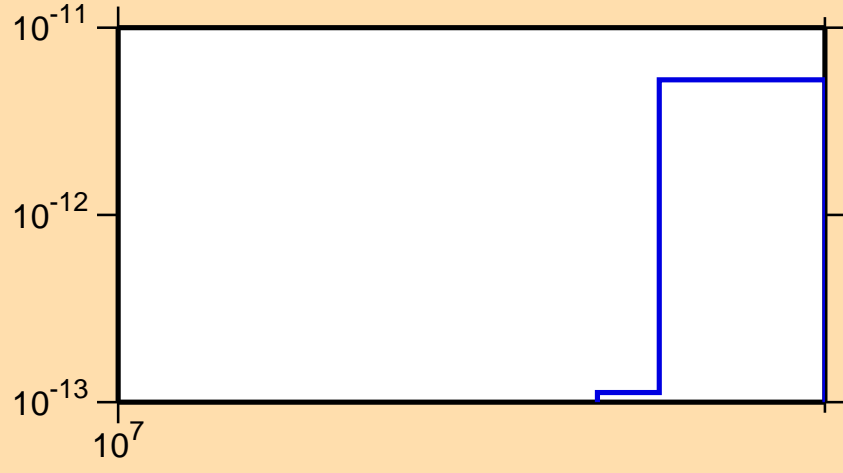
\sigma vs. E for ^{257}\text{Lw} (mt 34)
