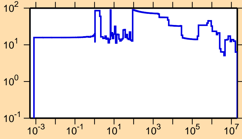
\Delta\sigma/\sigma vs. E for ^{257}\text{Lw}(n,el.)
