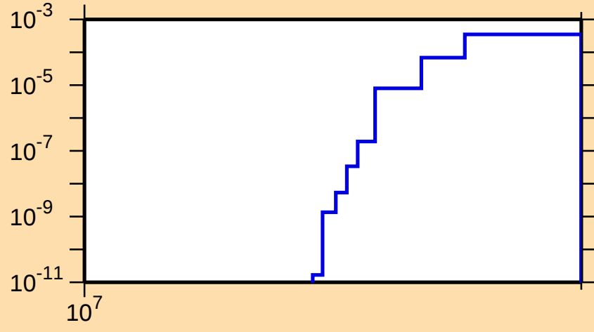
\sigma vs. E for ^{18}\text{Ne}(\text{mt } 34)
