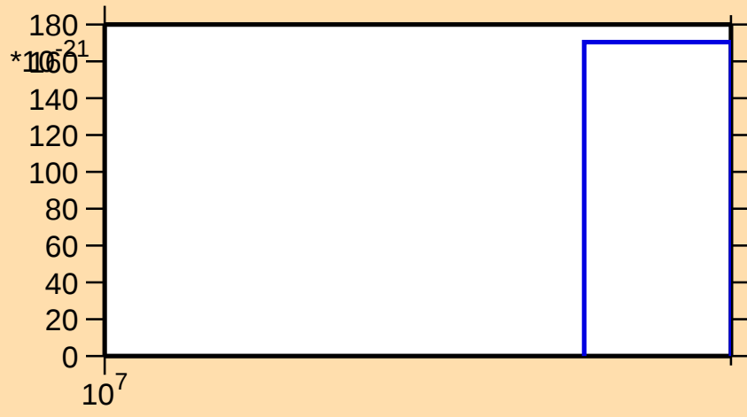
\sigma vs. E for ^{56}\text{Ni}(\text{mt } 34)
