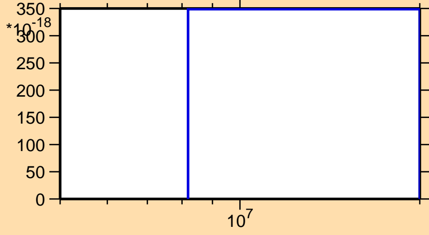
\sigma vs. E for ^{57}\text{Ni}(\text{mt } 45)
