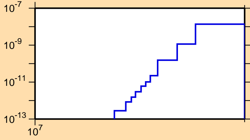
\sigma vs. E for ^{173}\text{Os} (mt 34)
