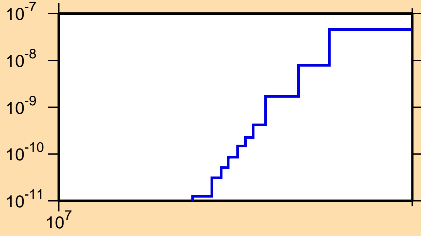
\sigma vs. E for ^{177}\text{Os} (mt 45)
