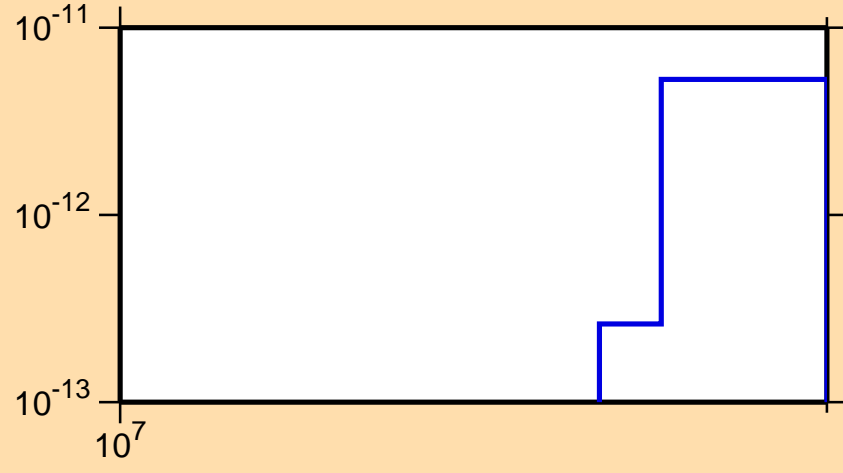
\sigma vs. E for ^{183}\text{Os} (mt 45)
