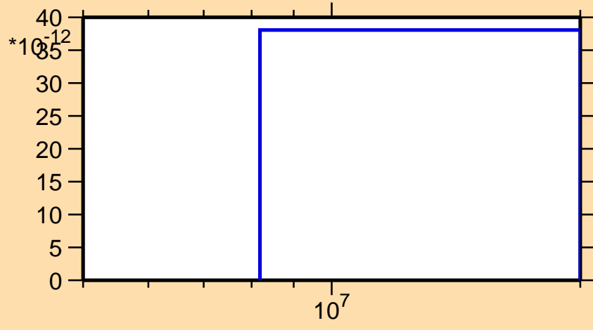
\sigma vs. E for ^{226}\text{Pa}(\text{mt } 45)
