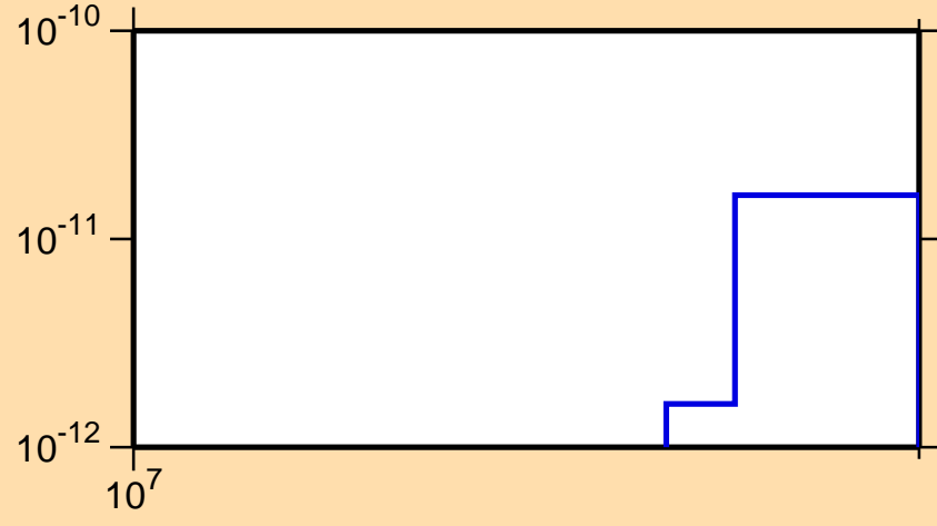
\sigma vs. E for ^{203}\text{Po}(\text{mt } 45)
