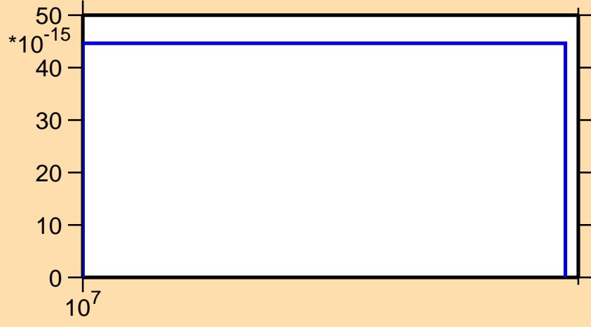
\sigma vs. E for ^{204}\text{Po}(\text{mt } 45)
