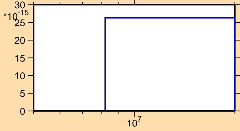
\sigma vs. E for ^{206}\text{Po}(\text{mt } 45)
