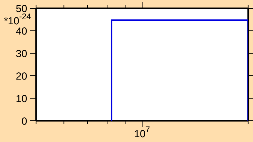
\sigma vs. E for ^{226}\text{Po}(\text{mt } 42)
