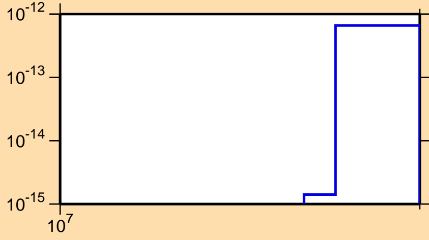
\sigma vs. E for ^{186}\text{Pt}(\text{mt } 34)
