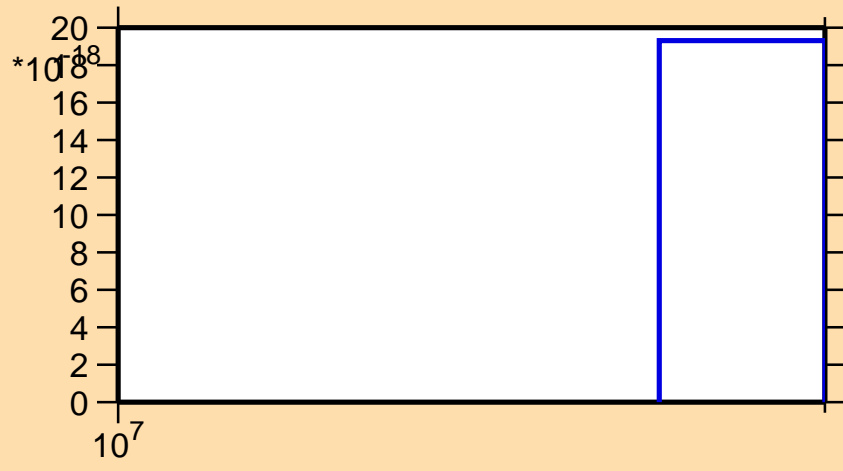
\sigma vs. E for ^{206}\text{Pt}(\text{mt } 42)
