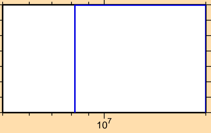
\sigma vs. E for ^{106}\text{Sn}(\text{mt } 45)
