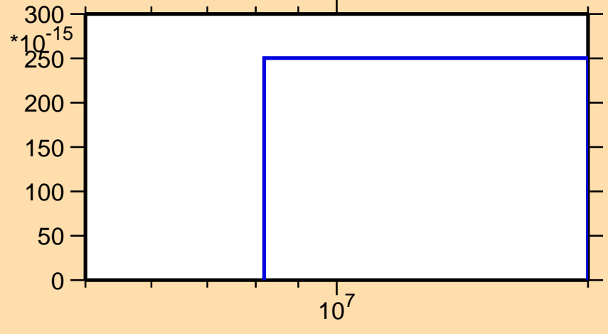
\sigma vs. E for ^{111}\text{Sn}(\text{mt } 34)
