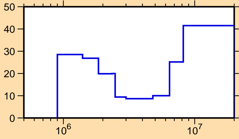
\Delta\sigma/\sigma vs. E for ^{179}\text{Ta}(n,incl.)
