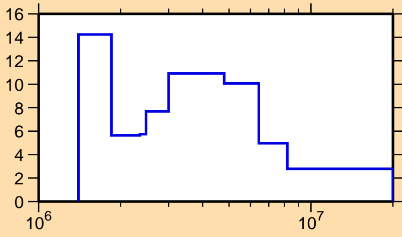
\Delta\sigma/\sigma vs. E for ^{183}\text{Ta}(n,tot.)
