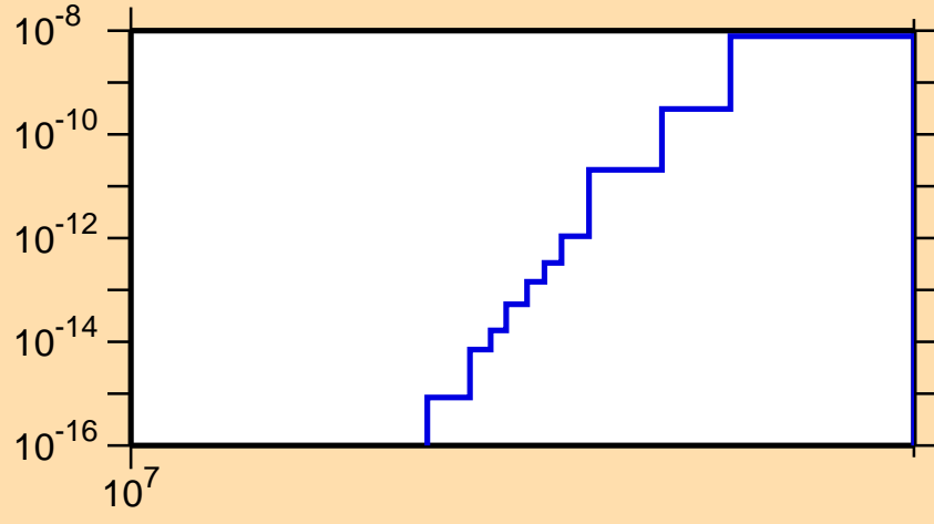
\sigma vs. E for ^{114}\text{Xe}(\text{mt } 34)
