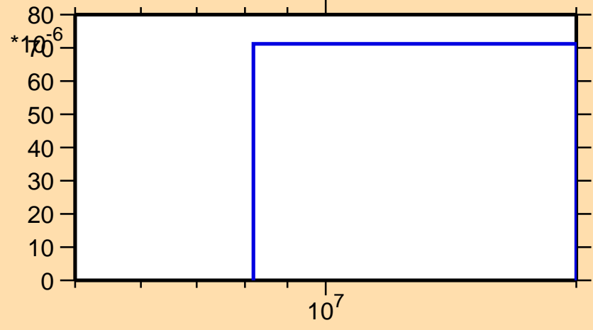
\sigma vs. E for ^{67}\text{As} (mt 45)
