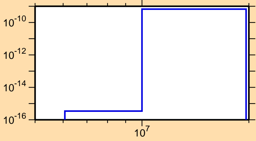
\sigma vs. E for ^{206}\text{At}(\text{mt } 45)
