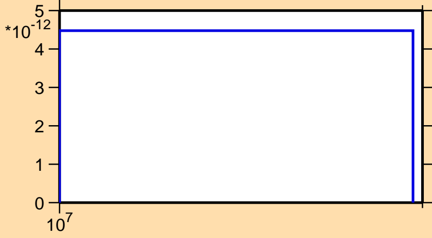
\sigma vs. E for ^{206}\text{At}(\text{mt } 34)
