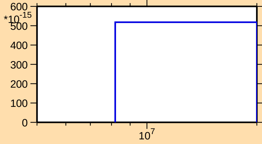
\sigma vs. E for ^{193}\text{Bi}(\text{mt } 34)
