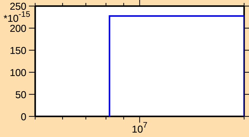
\sigma vs. E for ^{126}\text{Cs}(\text{mt } 34)
