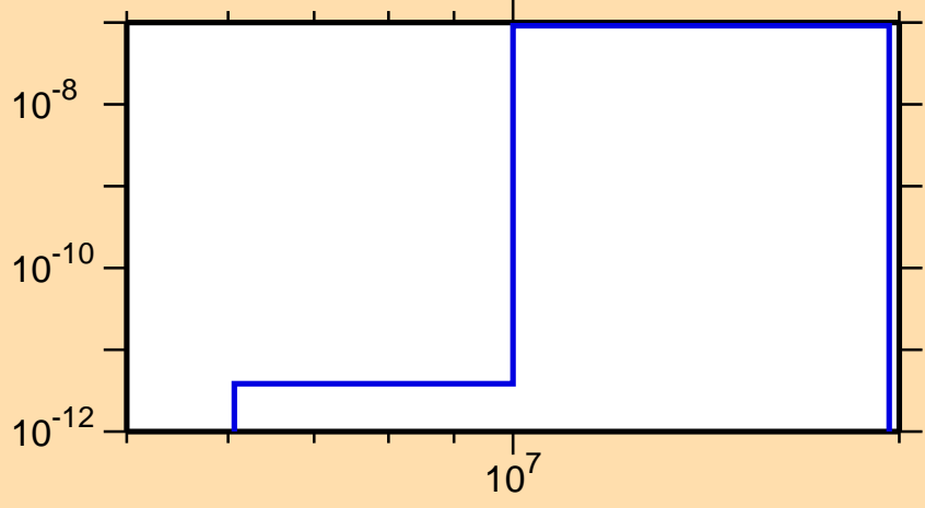
\sigma vs. E for ^{206}\text{Fr}(\text{mt } 45)
