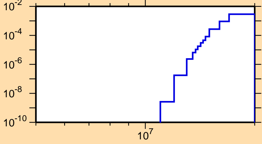
\sigma vs. E for ^{63}\text{Ga}(\text{mt } 45)
