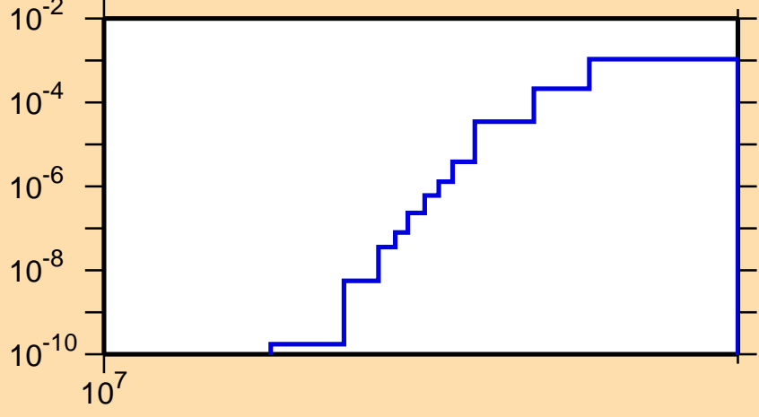
\sigma vs. E for ^{64}\text{Ga} (mt 45)
