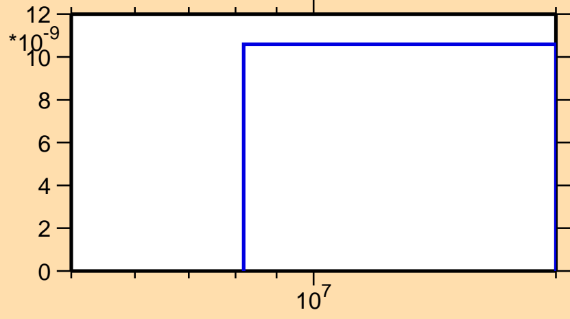
\sigma vs. E for ^{64}\text{Ga} (mt 34)
