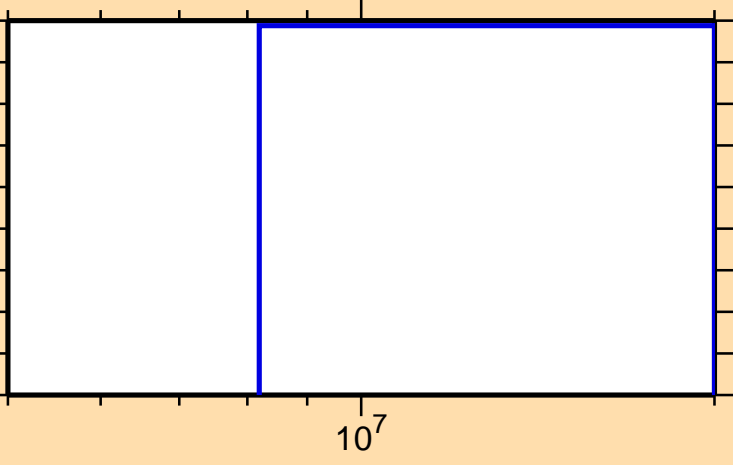
\sigma vs. E for ^{73}\text{Kr}(\text{mt } 34)
