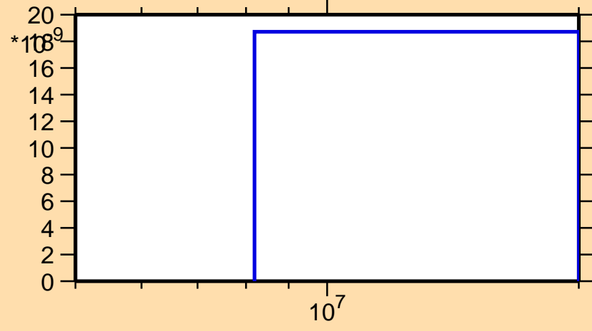
\sigma vs. E for ^{84}\text{Mo}(\text{mt } 45)
