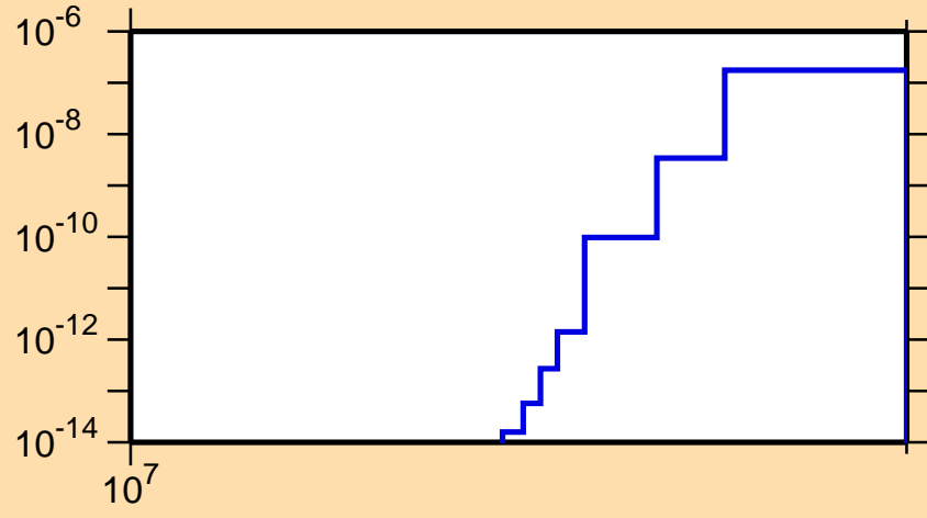
\sigma vs. E for ^{86}\text{Mo} (mt 45)
