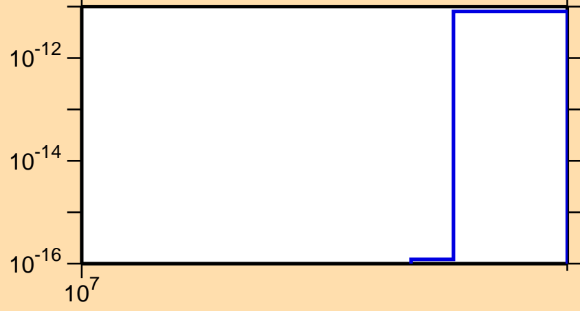
\sigma vs. E for ^{86}\text{Mo} (mt 34)
