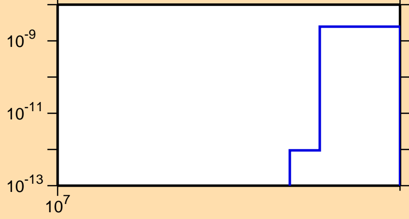
\sigma vs. E for ^{88}\text{Mo} (mt 45)
