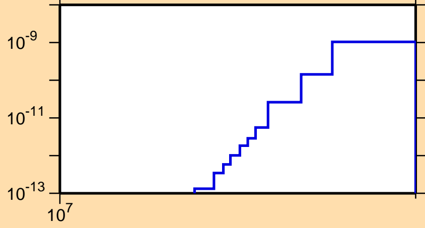
\sigma vs. E for ^{179}\text{Os} (mt 45)
